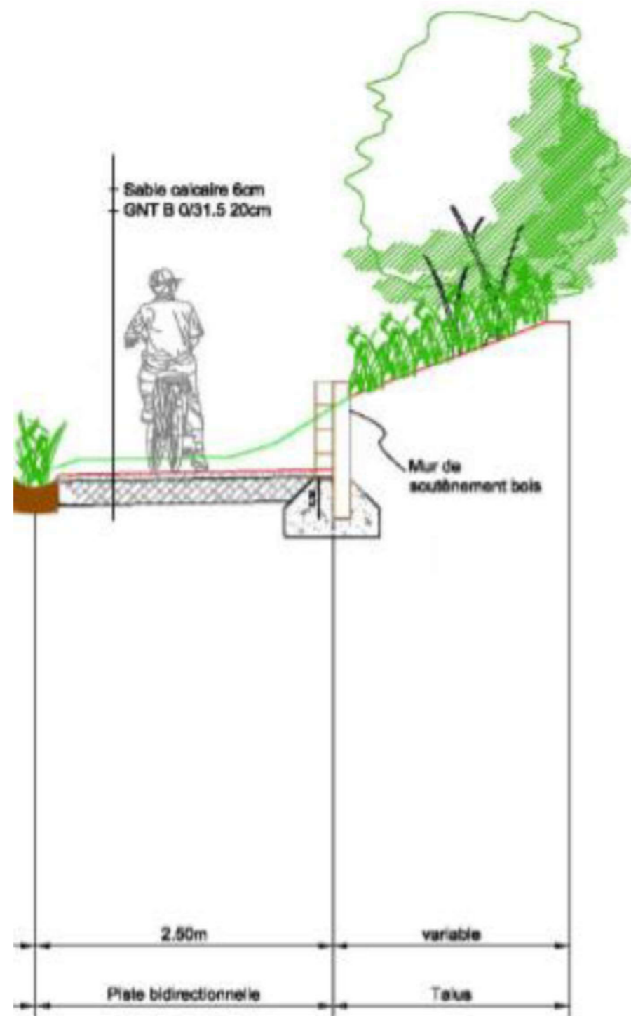
Figure 3 : Coupe type de site propre en milieu agricole ou naturel hors accotement
