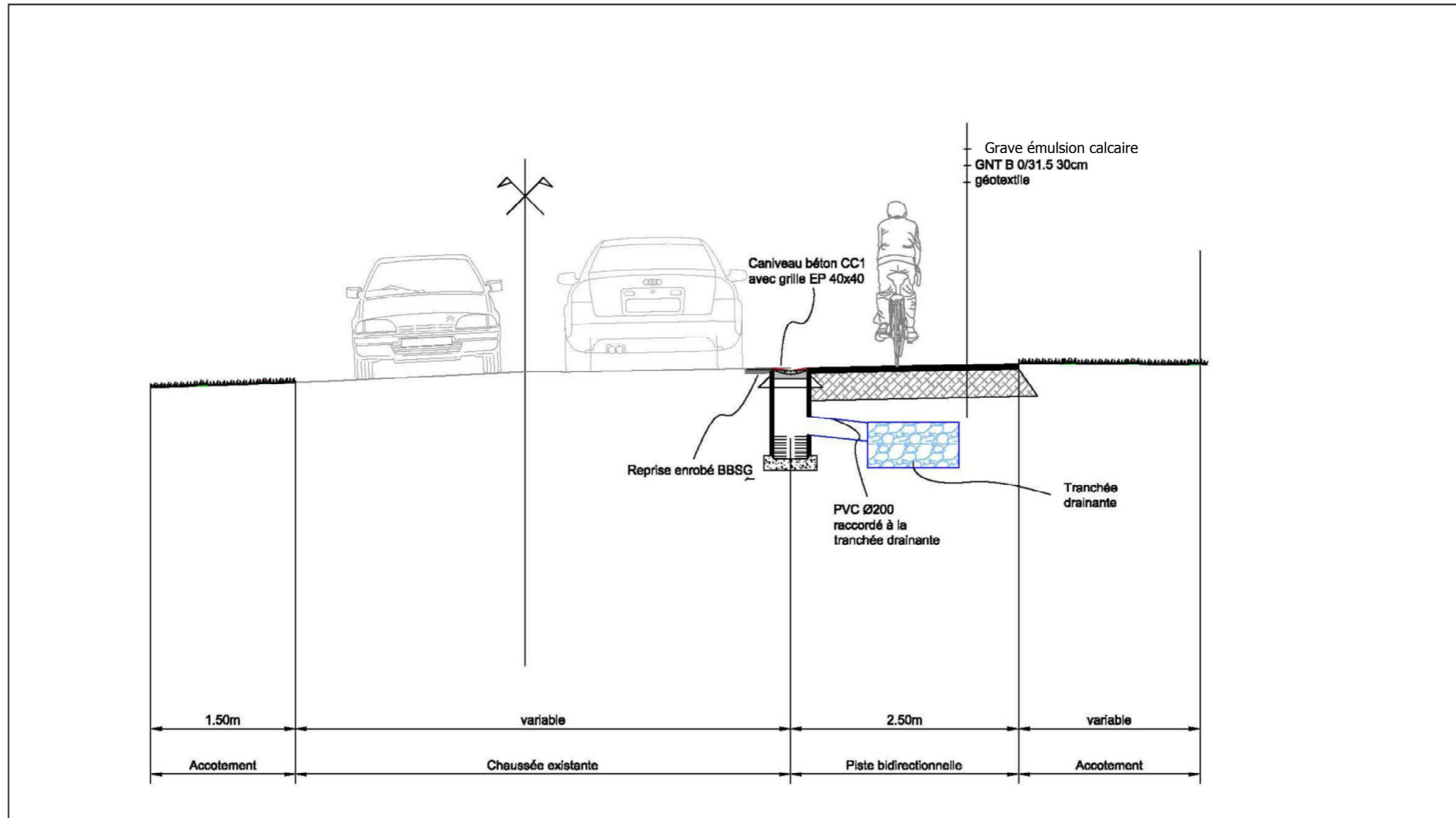
Figure 2 : Coupe type de site propre en milieu urbain ou accotement
